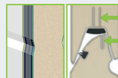
Remplissage panneaux acier à rupture de pont thermique et mousse isolante 40mm
