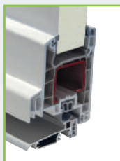
Profils PVC
